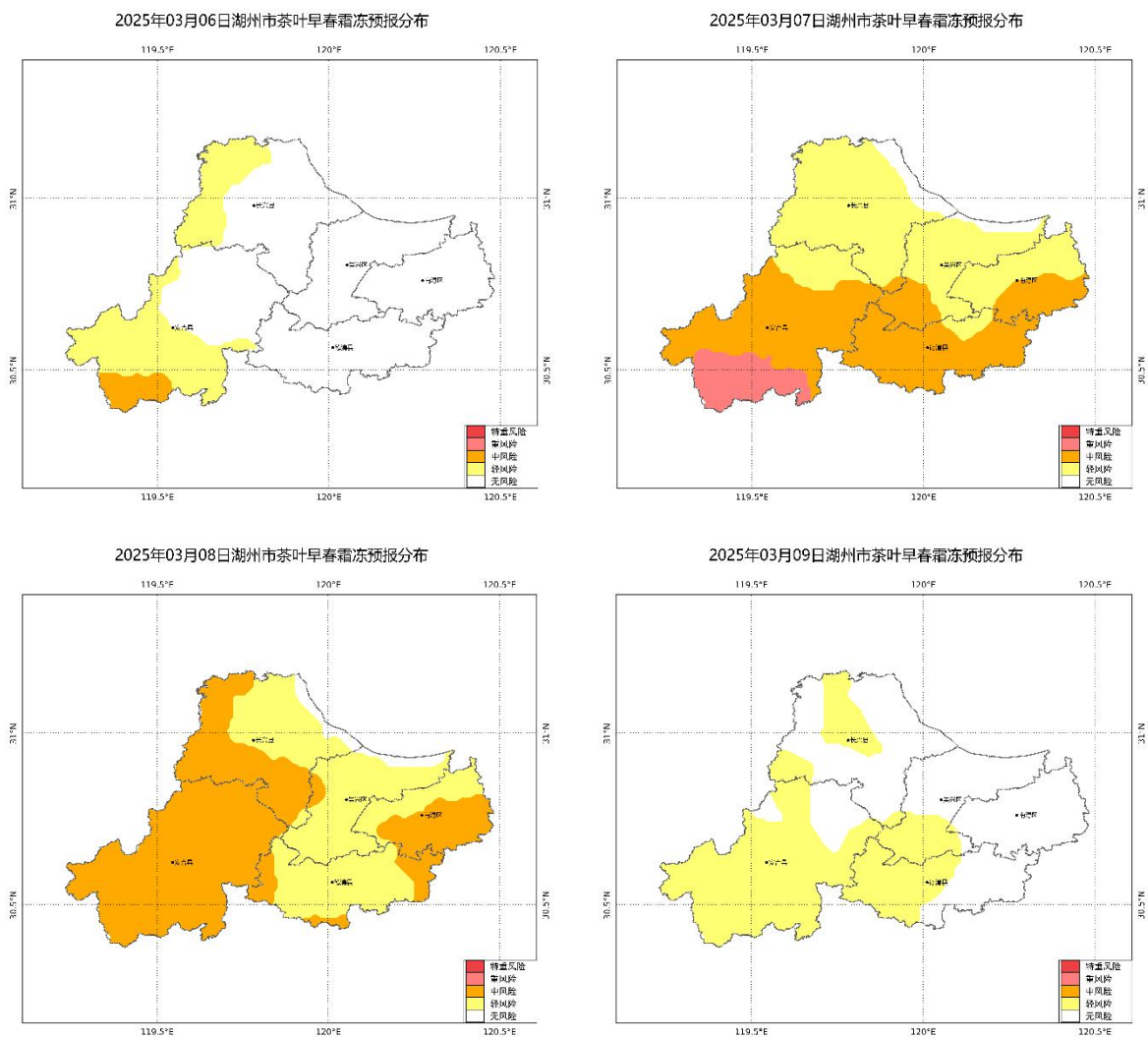
图2 2025年3月6-9日湖州市春茶霜冻害风险预警分布图
